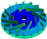
FEM of Flue Gas Fan Impeller
